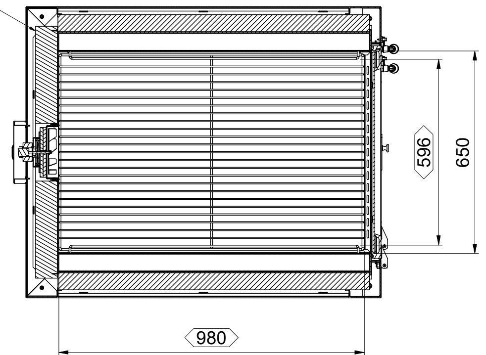
B-B ( 1 : 12 )
