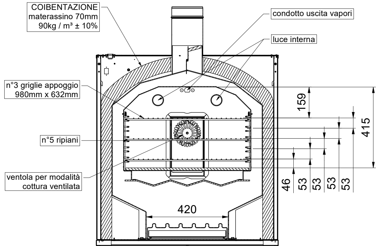
A-A ( 1 : 12 )
